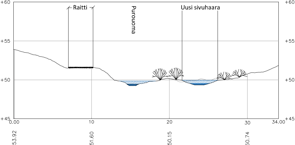
LEIKKAUS B-B'
