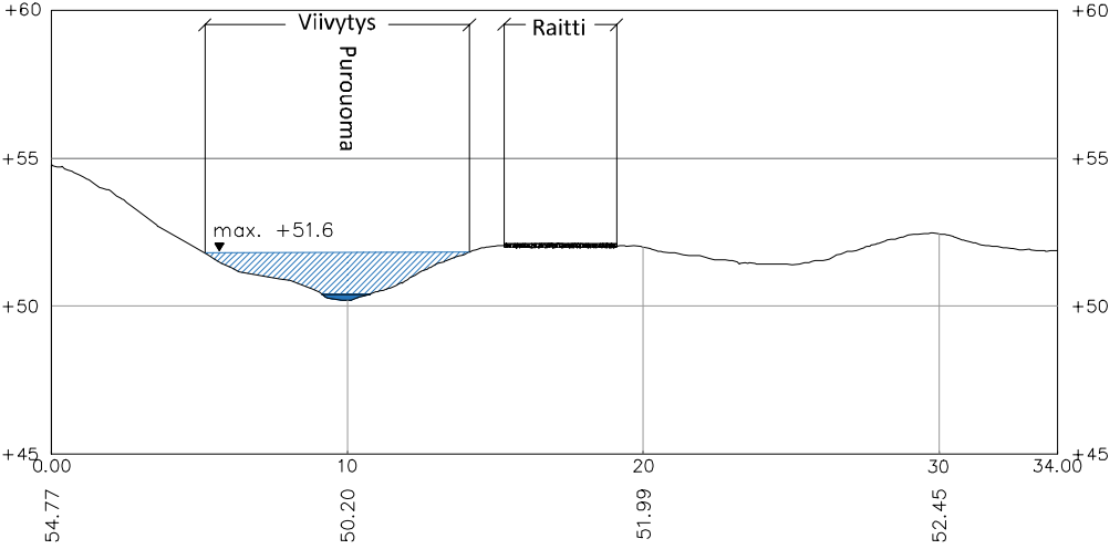
LEIKKAUS A-A'
